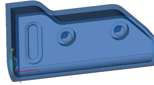
로컬 오프셋 미리 보기 바깥쪽
