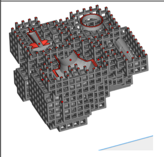
자유형 신터박스; 내부 벽; 적용됨
